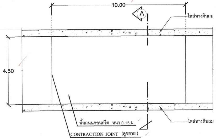
แปลนพื้นถนน คสล.
