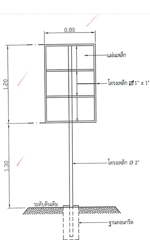
รูปด้านหลัง NOSCALE
