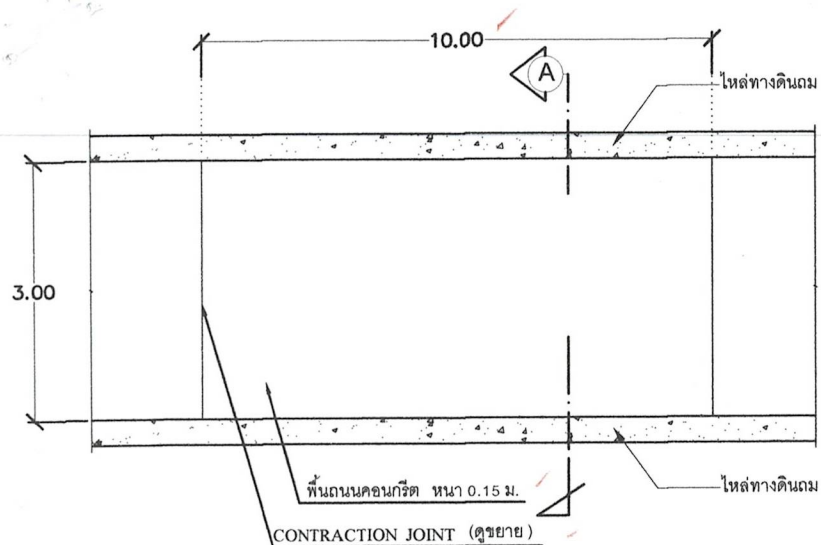
แปลนพื้นถนน คสล.
