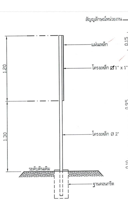
รูปด้านข้าง NOSCALE
