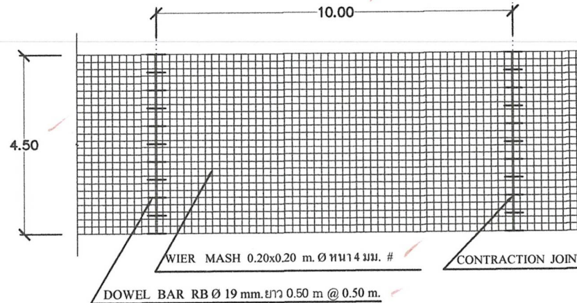
แปลนการเสริมเหล็กถนน คสล.
